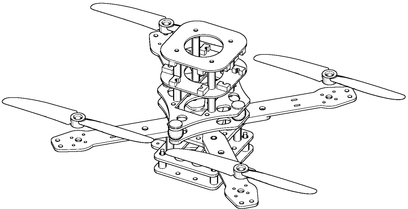
Seitenansicht FINken III
