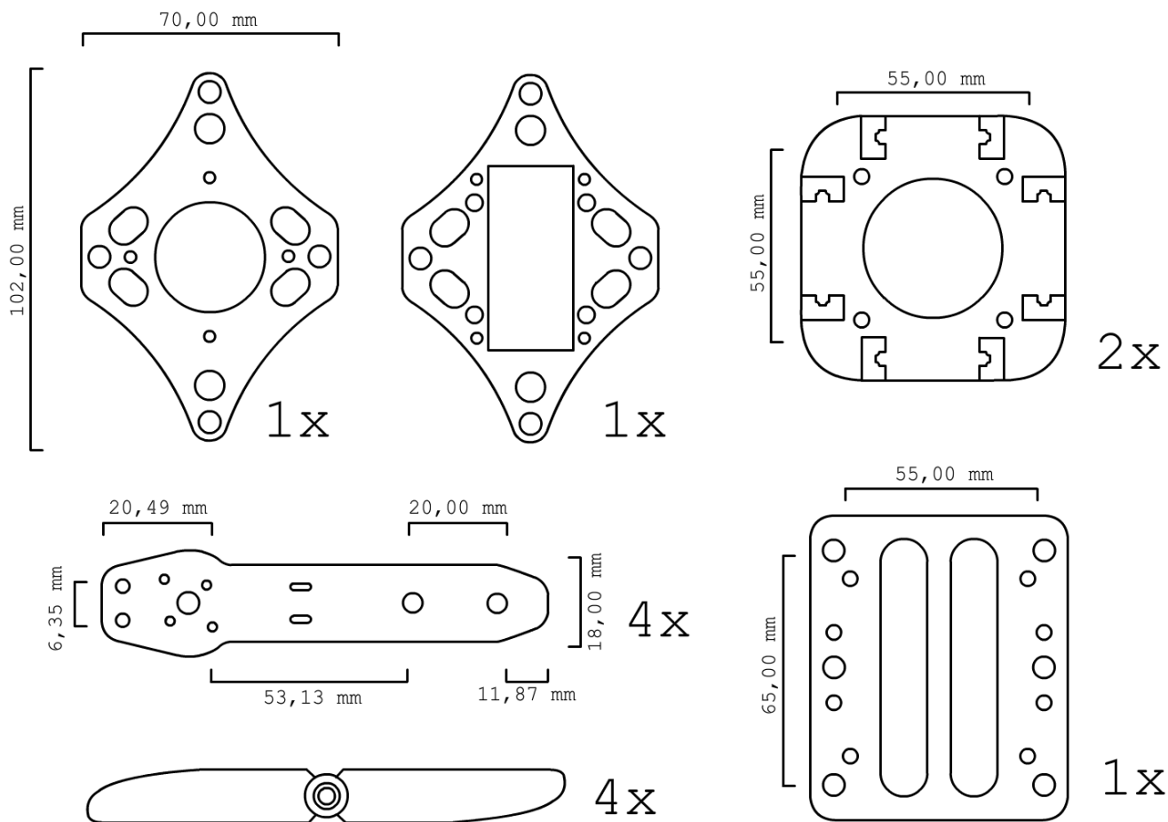
Bauteile FINken III
