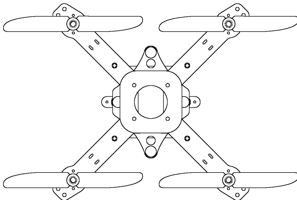
Aufsicht FINken III
